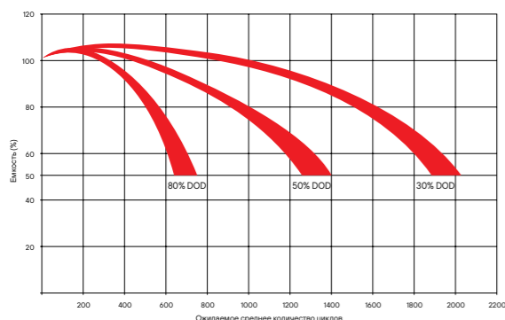
Циклический ресурс в зависимости от глубины разряда.
