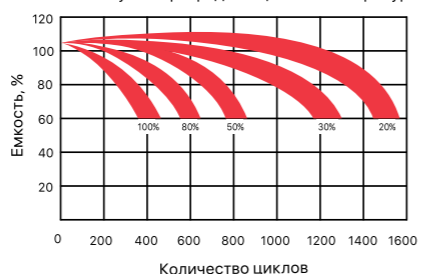
Влияние глубины разряда на циклический ресурс
