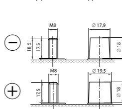
Двойной вывод DUAL
